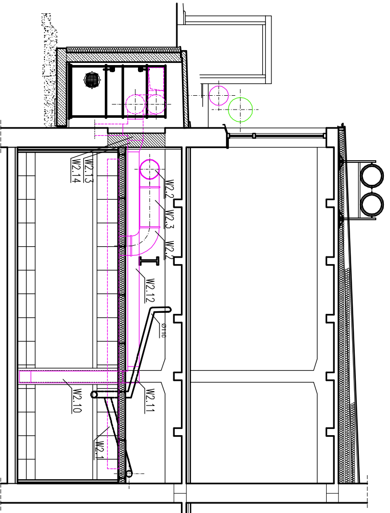
WIDOK B-B
